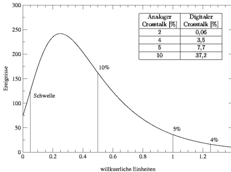
Abbildung 3.4: Die angenäherte Landauverteilung simuliert das Signalhöhenspektrum minimal ionisierender Teilchen. Die Signalhöhen, ab denen die Schwelle bei 10 %, 5% bzw. 4 % analogem Crosstalk überschritten werden, sind markiert. In der Tabelle ist der jeweils dazugehörige digitale Crosstalk eingetragen [24].
