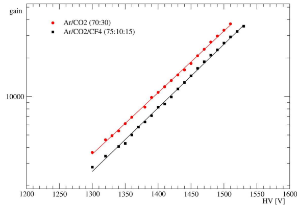
Abbildung 8.1: Die effektive Gasverstärkung in \text{Ar}/\text{CO}_2/\text{CF}_4 (75:10:15) und \text{Ar}/\text{CO}_2 (70:30) aufgetragen über die Betriebsspannung.
