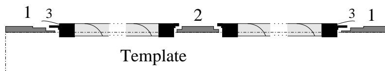
Abbildung 2.24: Längsschnittskizze durch das bestückte Template. Die HV-Durchführungsplatinen (1) und die Mittelplatine (2) sind auf dem Template positioniert. Die einzelnen Strawtubes werden in das Template eingelegt, wobei ihre Endstücke an die Stufen der Platinen gesetzt werden. Die Fähnchen der Strawtubes (3) werden an die Massenkontakte der HV-Durchführungsplatinen (1) gelötet.
