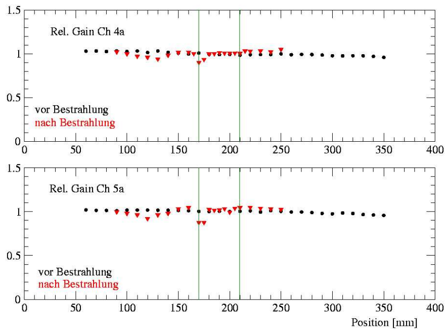
Abbildung 6.14: Die relative Gasverstärkung entlang der bestrahlten Strawtubes bei 500 ppm Wasser in \text{Ar}/\text{CO}_2 , vor und nach der Bestrahlung. Die bestrahlte Region entlang der Kanäle erstreckt sich über 4 cm von Position 170 bis 210 und ist durch die Linien markiert. Position 0 entspricht dem unteren, Position 400 dem oberen Ende des Moduls. Die Gasflussrichtung war in Richtung Position 400.
