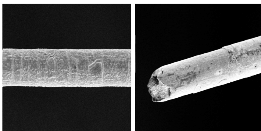
Abbildung 7.10: REM-Aufnahmen bestrahlter Anodendrähte aus der mit Ar/CO 2 /CF 4 betriebenen Kammer. Links ist ein Ausschnitt des Drahtes aus Kanal 3b zu sehen. Rechts ist der gerissene Draht aus Kanal 4b gezeigt.
