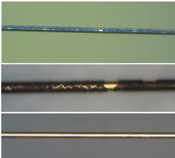
Abbildung 7.9: Bestrahlte Stellen von Anodendrähten unter dem Lichtmikroskop betrachtet. Oben: Draht aus Kanal 3b (mit Drahtpositionierer), betrieben in Ar/CO 2 /CF 4 . Mitte: Draht aus Kanal 4b (ohne Drahtpositionierer), betrieben in Ar/CO 2 /CF 4 . Der Draht riss während des Betriebs. Unten: Draht aus Kanal 5a (in Ar/CO 2 betrieben). An ihm sind keine Unterschiede zu einem neuen Draht zu sehen.
